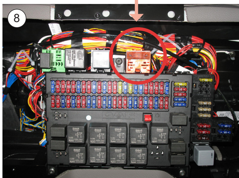
Maxi-fusible 40 A
